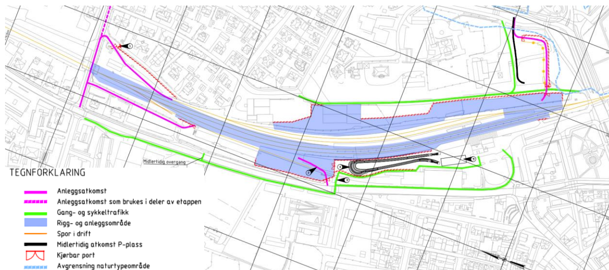
Figur 4-14: Illustrasjon underbygningsetappe 2
