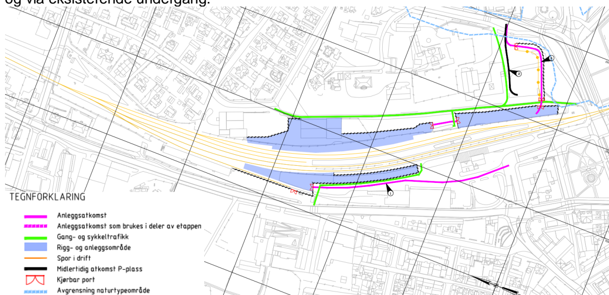
Figur 4-13: Illustrasjon underbygningsetappe 1
