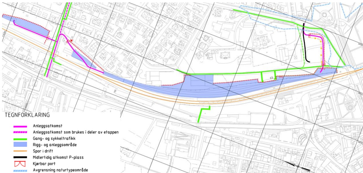
Figur 4-17: Illustrasjon underbygningsetappe 5
