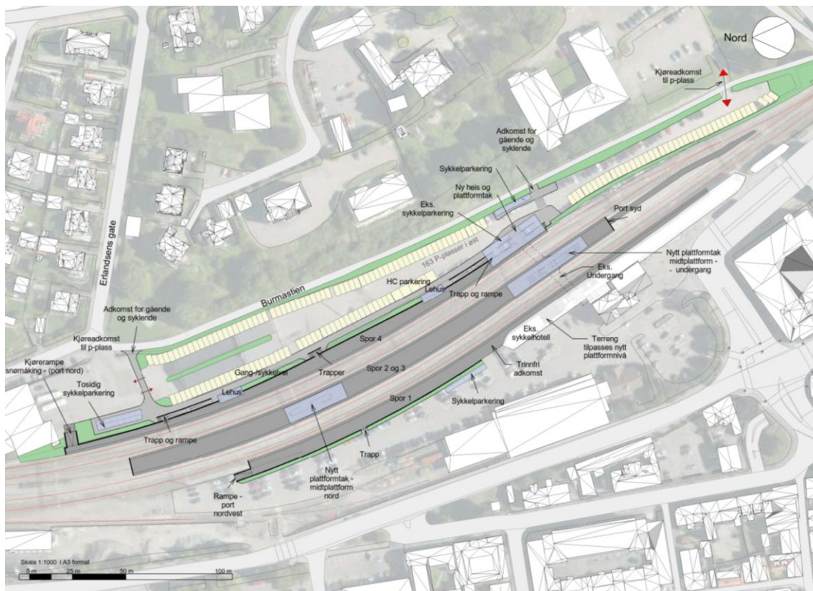
Figur 4-2: Oversiktstegning av stasjonsområdet med fire spor til plattform, ny østre plattform og oppgradering av eksisterende plattformer.
