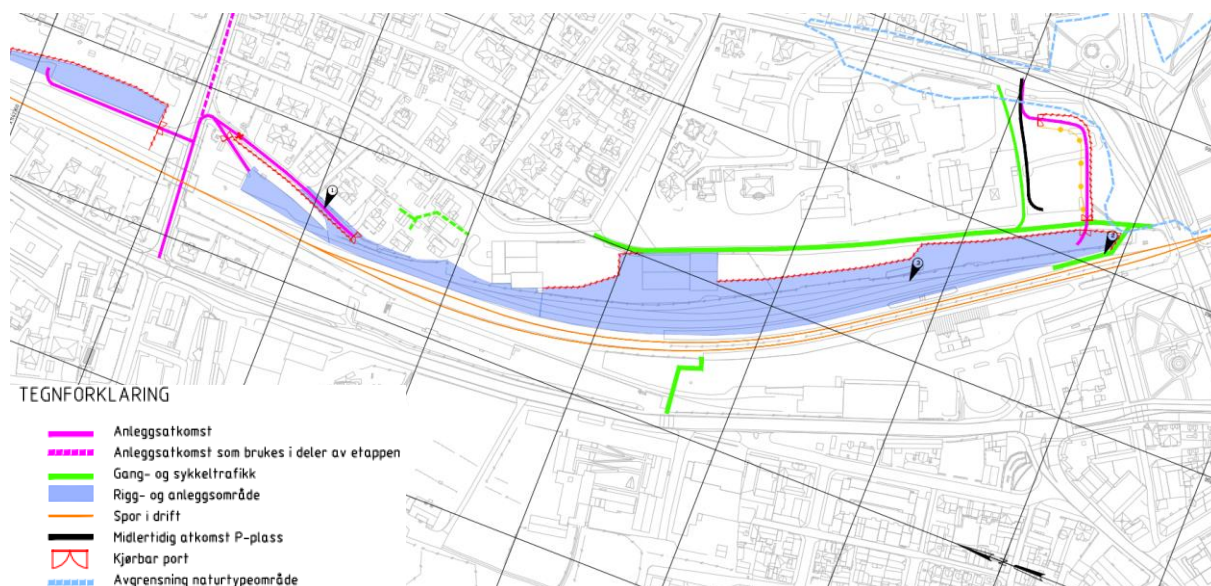
Figur 4-15: Illustrasjon underbygningsetappe 3
