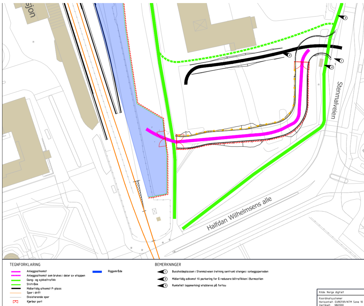
Figur 6-3: Midlertidig atkomst/kryss i Stenmalveien i anleggsperioden
