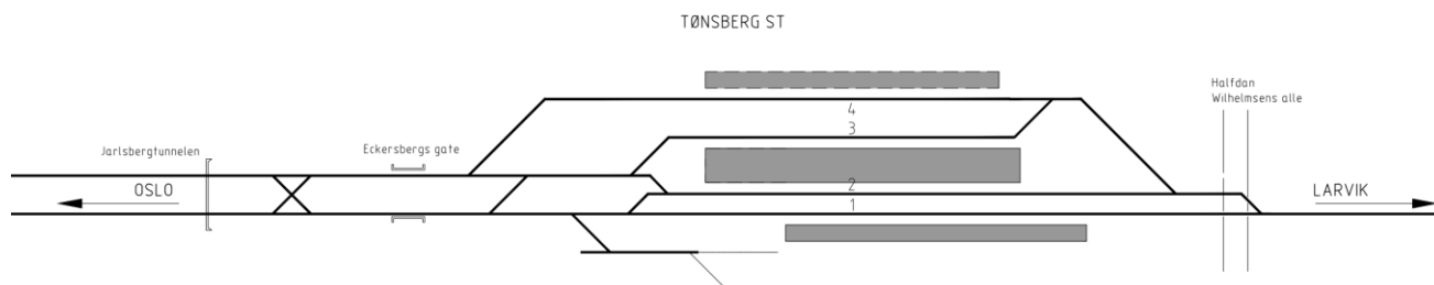
Figur 4-1: Skjematisk sporplan Tønsberg stasjon
