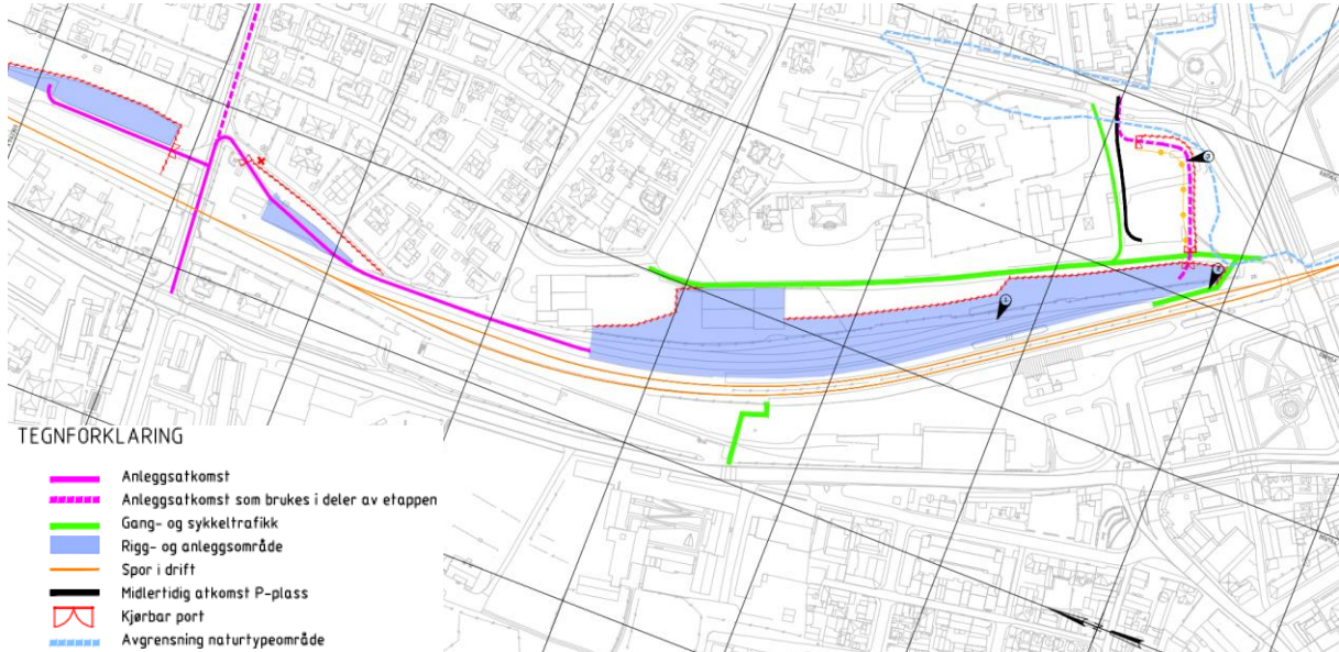
Figur 4-16: Illustrasjon underbygningsetappe 4
